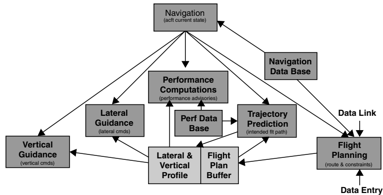
Figura 11: Diagrama de Bloco das Principais Funções do Computador de Bordo
