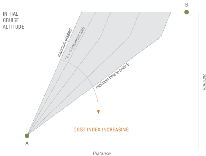
Gráfico 12: Variações do Cost Index para Climb Fonte: Boeing 2007
